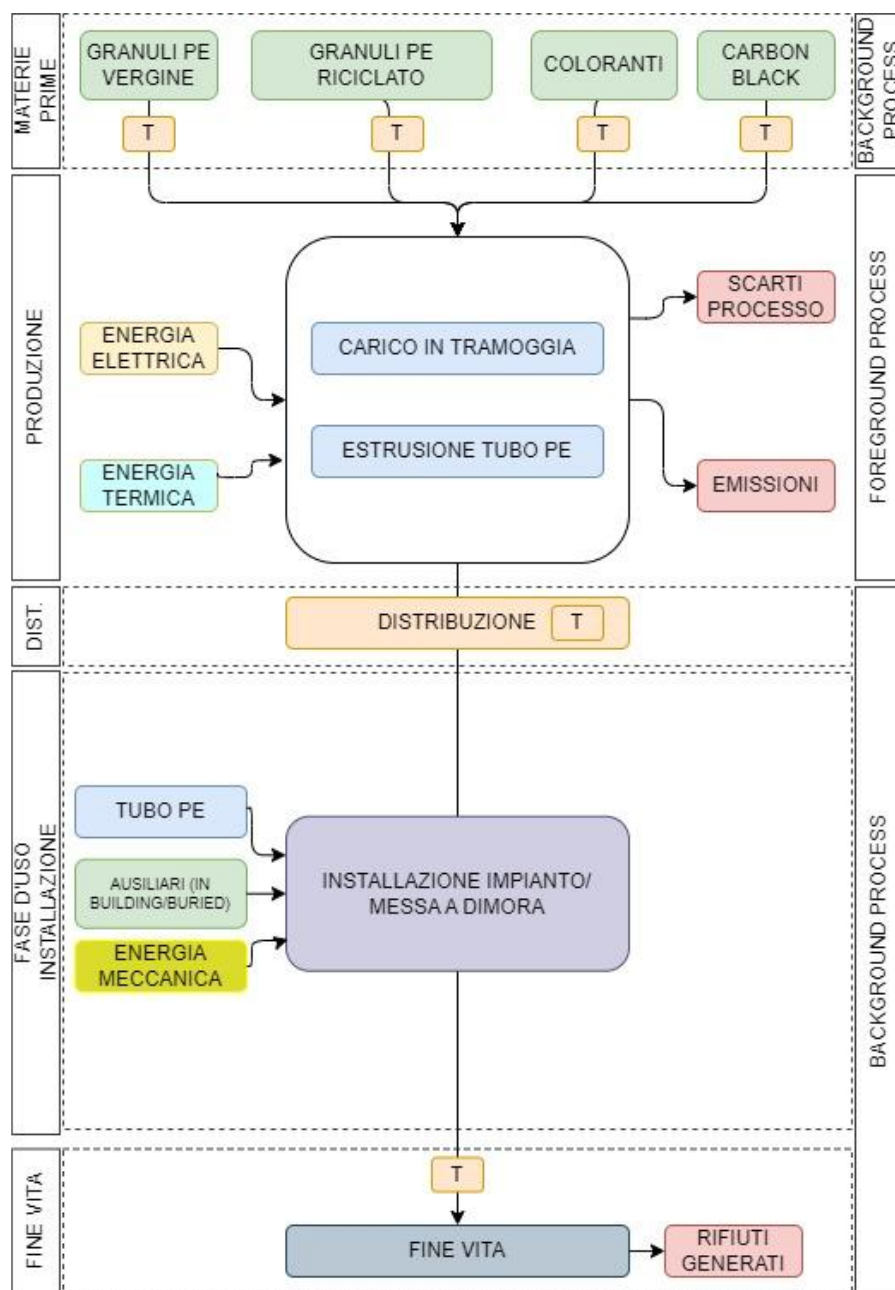
Figura 3 - Diagramma dei confini del sistema per le tubazioni in PE per il trasporto di fluidi oggetto di studio (Prodotti rappresentativi 1 e 2)
