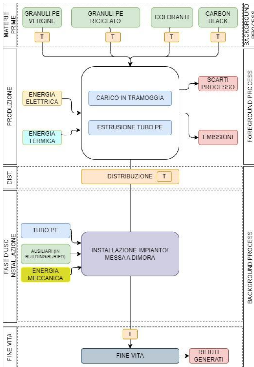
Figura 2 - Diagramma dei confini del sistema per le tubazioni in PE per il trasporto di fluidi oggetto di studio (Prodotti rappresentativi 1 e 2)
